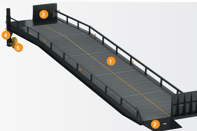
Рампа мобильная с трехсторонней загрузкой серии 3SRM
